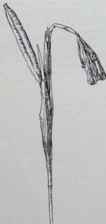
FIG. 27. Spathes and capsule of I. xiphium .
